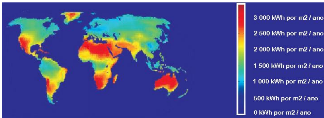
Figura 01 - Radiação direta normal
